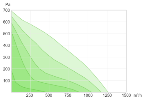
VKAP 315 LD
