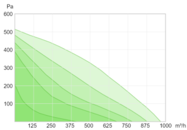
VKAP 250 LD
