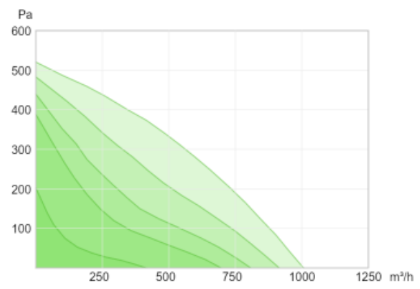
VKAP 200 LD
